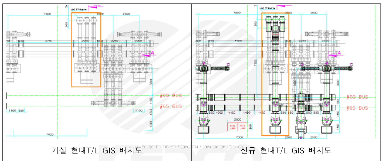
[그림1] 음성S/S 154kV 현대T/L GIS 기기배치방안
